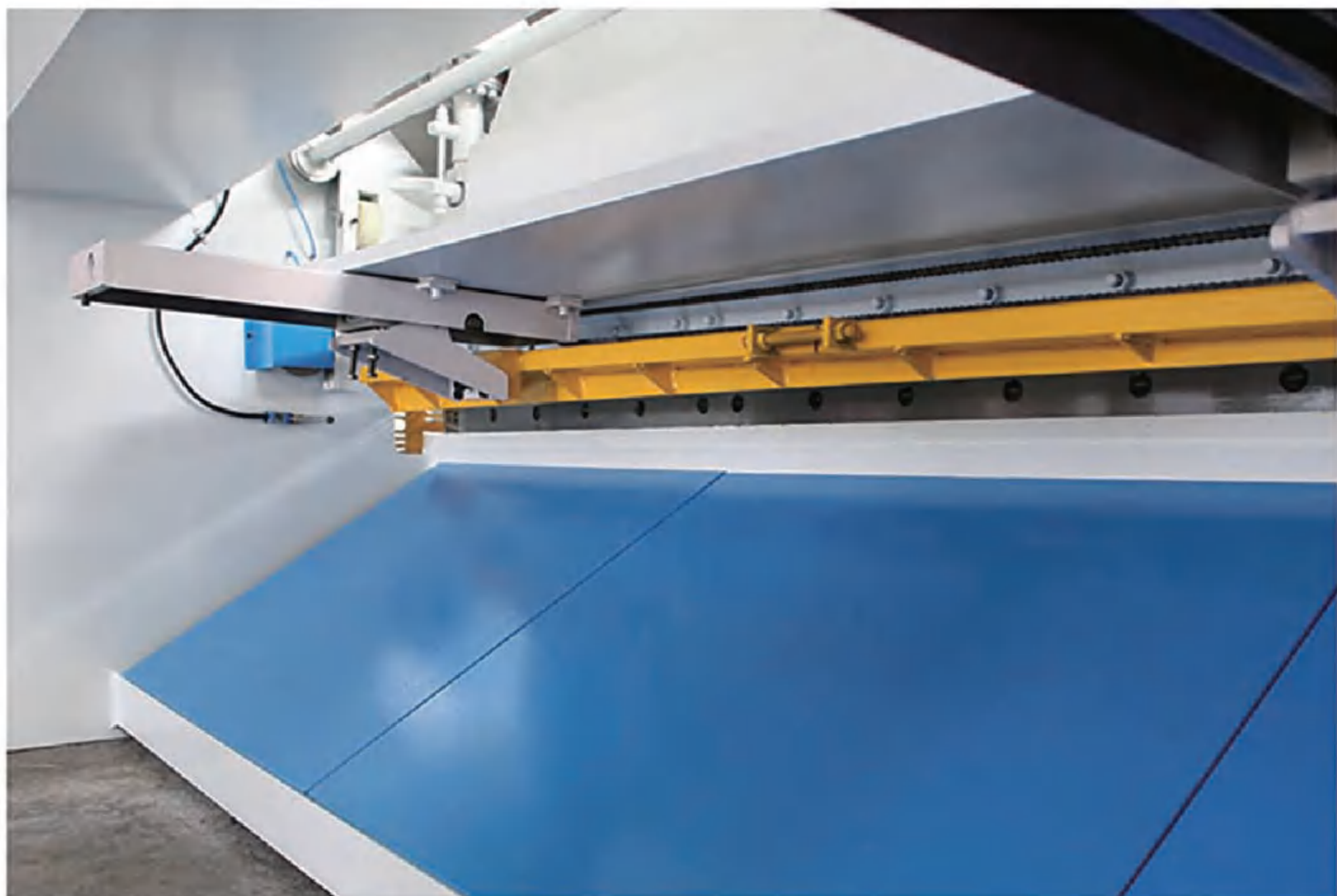
Задний упор высокой точности
