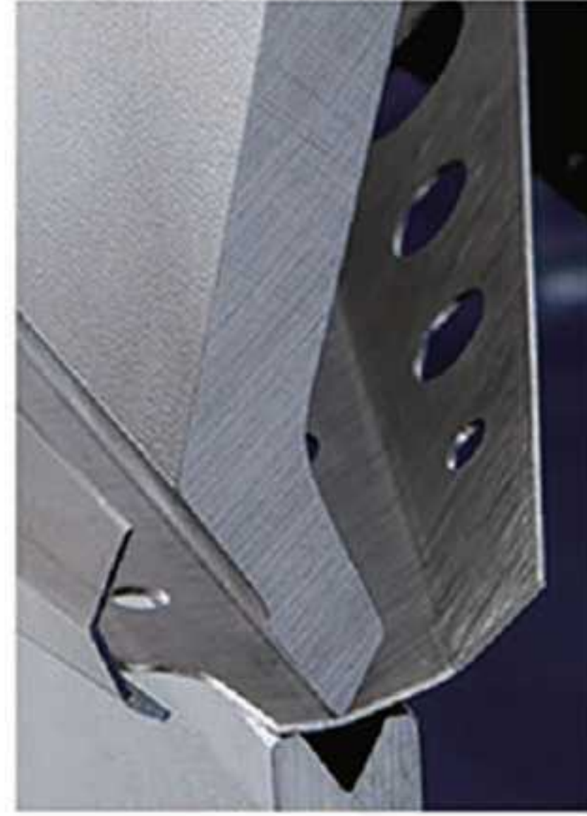
Схема гибки
